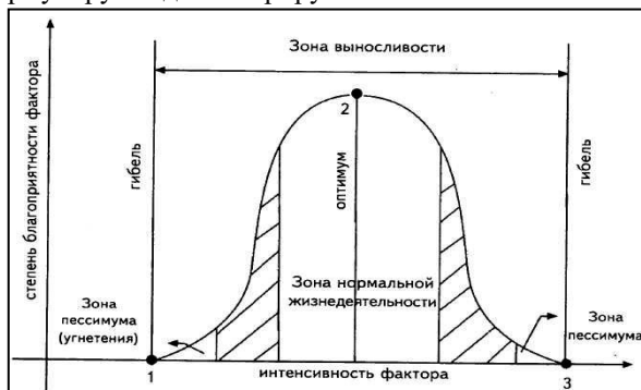
Рис.2. Общая схема действия экологического фактора на живой организм
